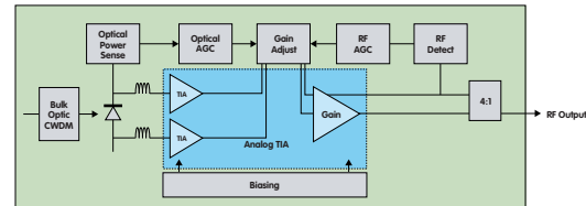
FTTH / RfOG
