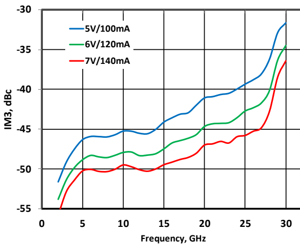
Figure 54 - IM 3 vs. V DD /I DD , 10dBm(per tone)
