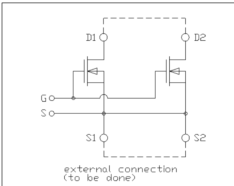
Single SiC MOSFET Module 240 Amperes / 10kV
