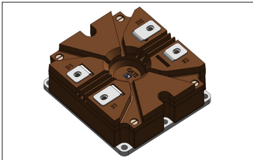
Single SiC MOSFET Module 240 Amperes / 10kV
